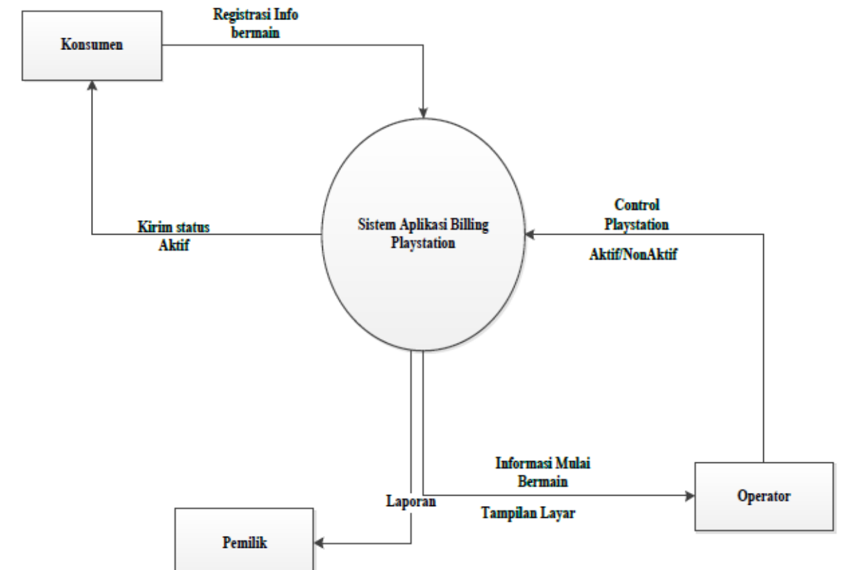
Gambar 2. Diagram Konteks
